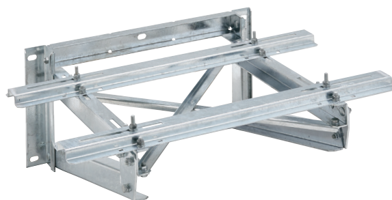
壁面用ブラケットタイプ
